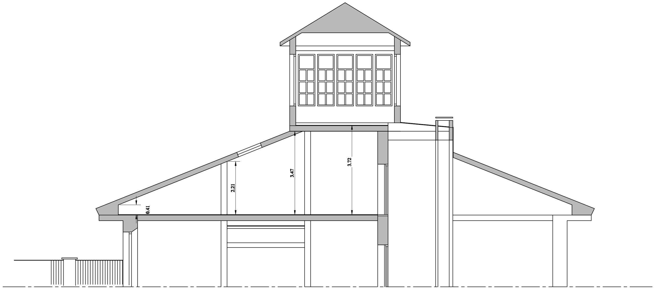
Sección A-B
